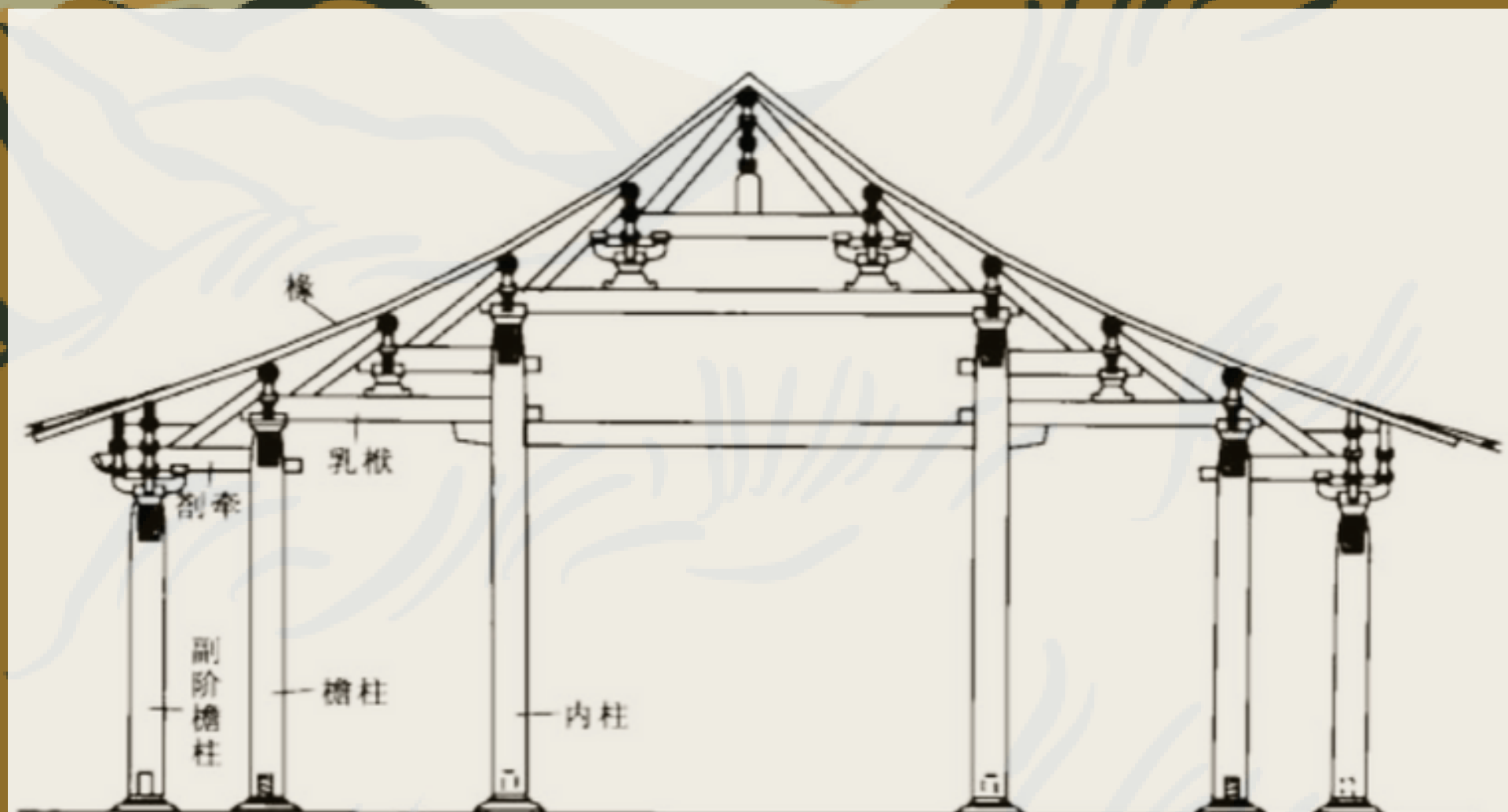
图1-216 十架椽屋前后各剖牵乳楹用六柱
